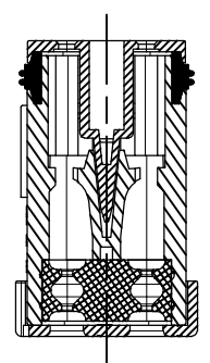
A-A
